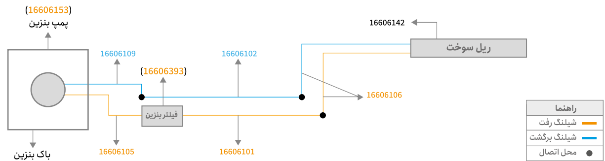
سیستم سوخت رسانی پیکان و وانت انژکتور (این تانک) مدل ۸۴ - ۸۵
