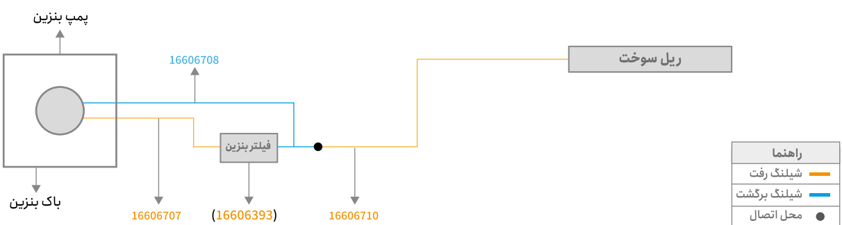
سیستم سوخت رسانی پراید انژکتوری یورو ۴
