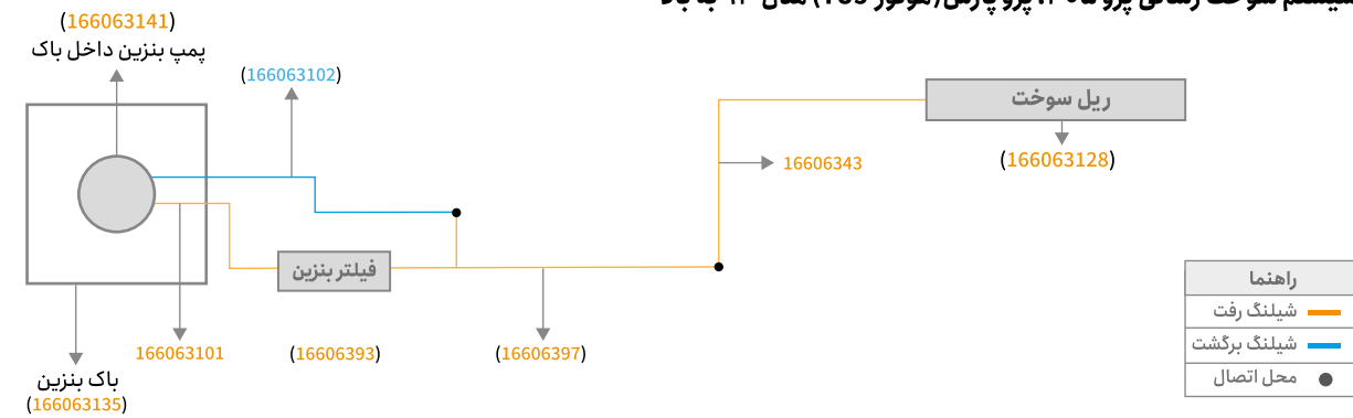
سیستم سوخت رسانی پژو پارس ELX (موتور زانتیا) مدل ۸۰ - ۸۲ - ۸۳ - ۸۴
