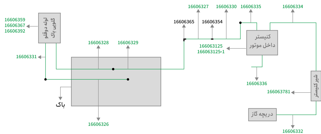
سیستم شیلنگ‌های بخار بنزین 405 و سمند تا مدل ۱۳۹۴
