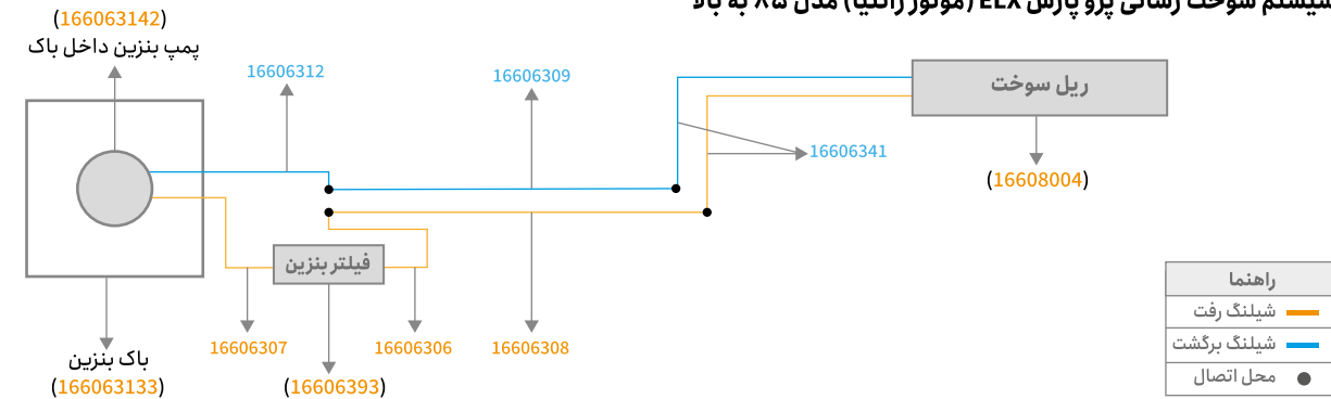
سیستم سوخت رسانی پژو پارس ELX (موتور زانتیا) مدل ۸۵ به بالا
