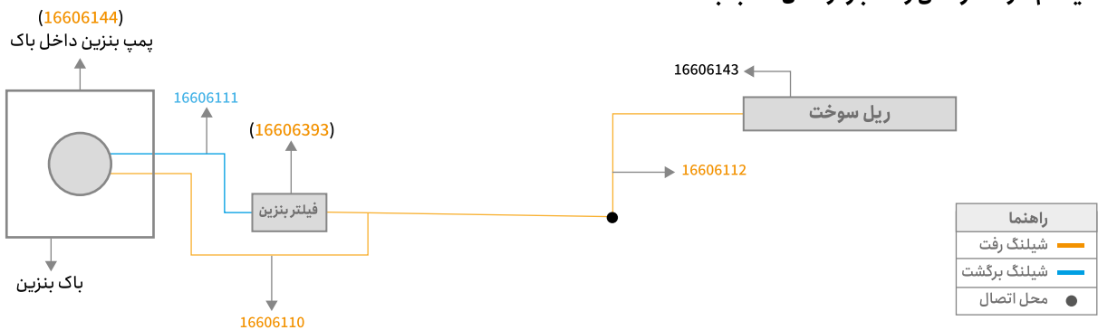
سیستم سوخت رسانی وانت باردو مدل ۸۶ به بالا
