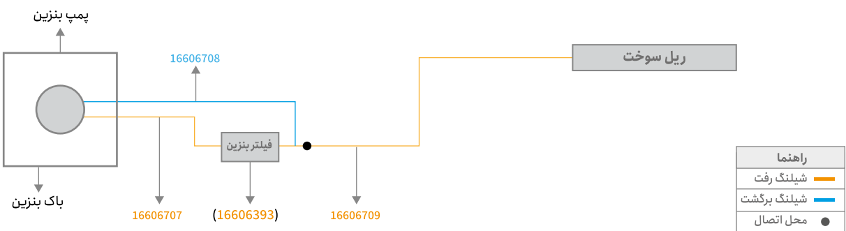
سیستم سوخت رسانی پراید انژکتور مدل ۹۰ تا ۹۴
