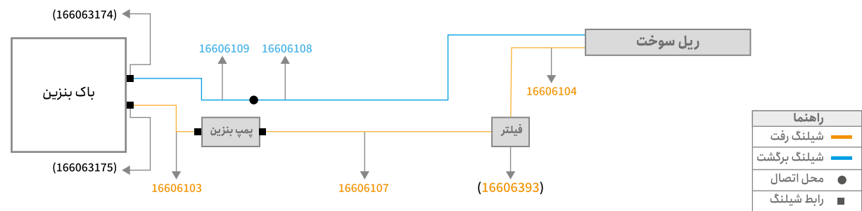
سیستم سوخت رسانی پیکان و وانت انژکتور (این تانک) مدل ۸۴ - ۸۵
