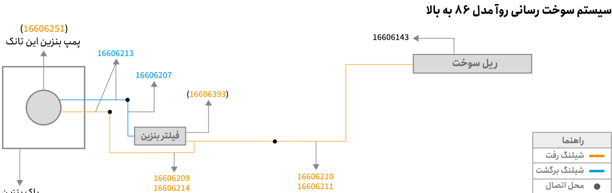
سیستم سوخت رسانی وانت آریسان مدل ۹۴ به بالا
