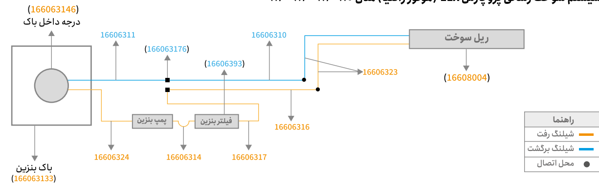
سیستم سوخت رسانی پژو پارس ELX (موتور زانتیا) مدل ۸۵ به بالا
