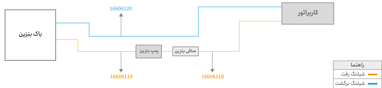
سیستم سوخت رسانی پیکان و وانت انژکتور (این لاین) مدل ۸۰ تا ۸۳
