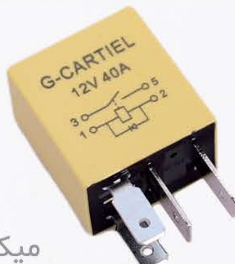
رله زرد 4 فیش کتابی
